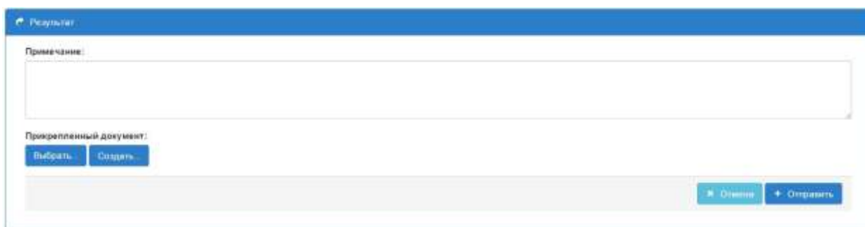
Рисунок 10 - Окно «Результат»
